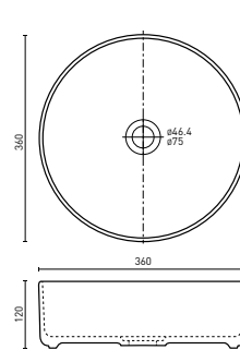
FLORENCIA - Round (p. 50 & 51) 360 x 360 x 120 (7L)
