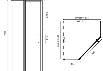
PREZZO (P. 38) 900 x 900 x 2000 mm
