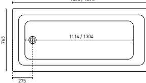
ARIA (P. 16) 1525 x 765 x 475 mm (138L) 1675 x 765 x 475 mm (156L)
