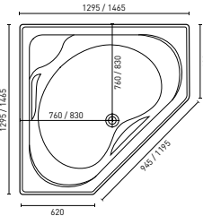
ANGELIQUE (P. 16) 1295 x 1295 x 480 mm (179L) 1465 x 1465 x 480 mm (259L)
